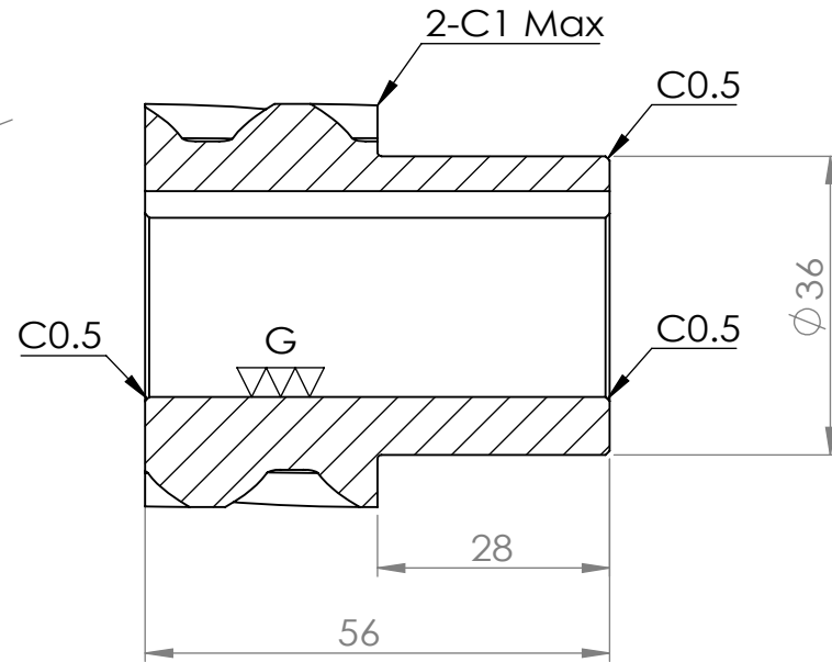
剖面圖 A-A
